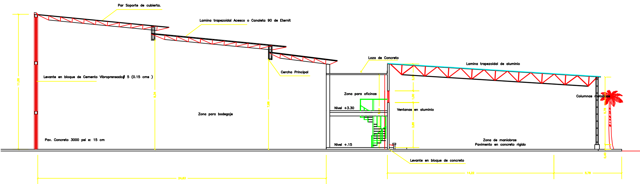
Corte transversal
